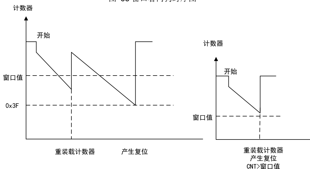
图 65 窗口看门狗时序图
