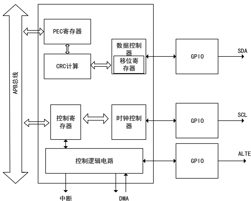
图 78 I2C 功能结构图
