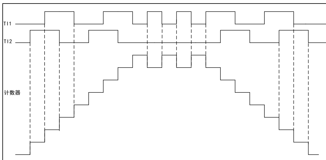
图 40 编码器模式下的计数器操作实例
