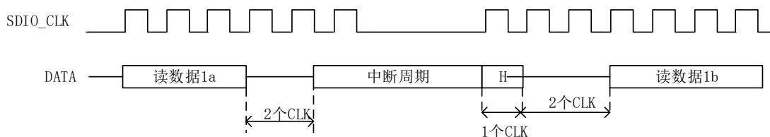
图 126 通过停止 SDIO_CLK 的读等待操作
