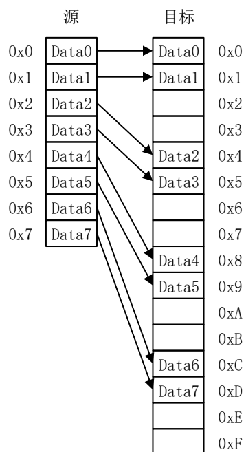
图 16 源为 16bits 目标为 32bits 的传输宽度
