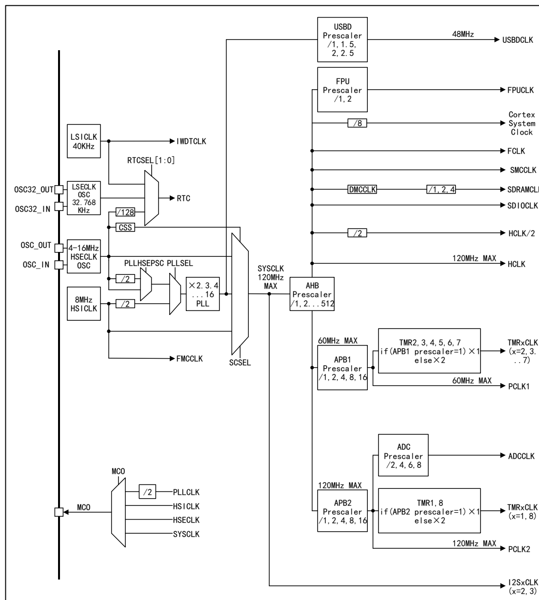
图 7 APM32E103xCxE 时钟树
