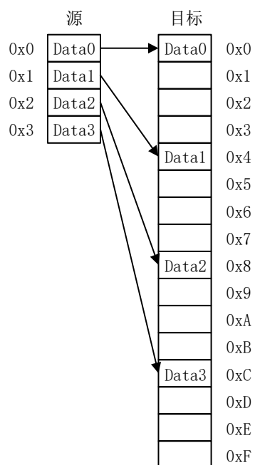
图 13 源为 8bits 目标为 32bits 的传输宽度
