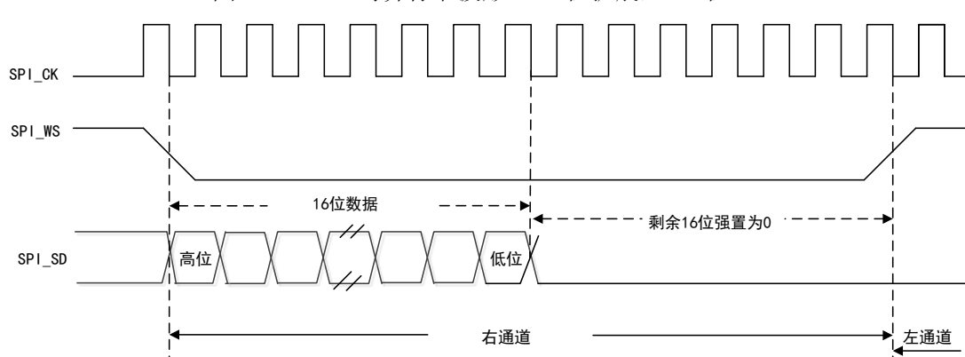
图 104 MSB 对齐标准波形（16 位扩展至 32 位）
