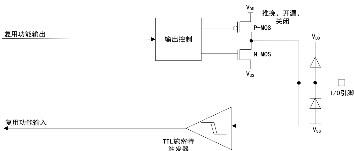
图 23 复用模式 I/O 结构
