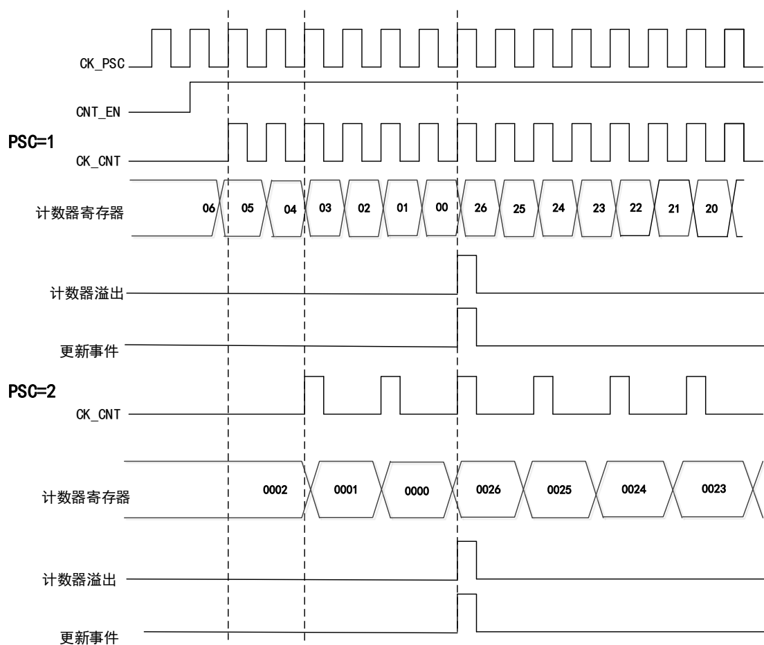
图 47 向下计数模式下，分频因子为 1 或 2 的时序图
