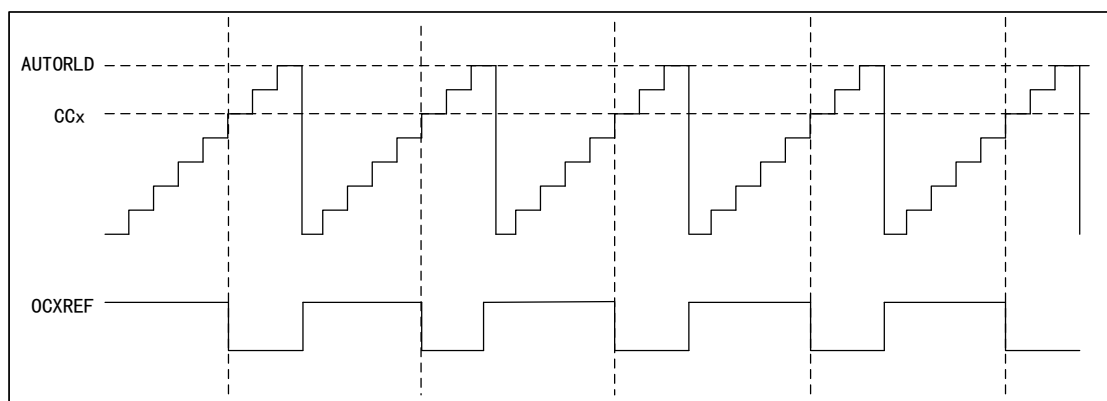
图 29 PWM1 向上计数模式的时序图
