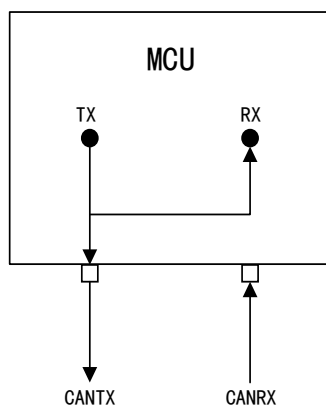
图 113 CAN 工作在环回模式
