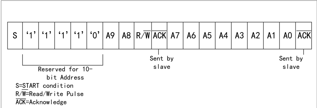
图 88 10 位地址格式
