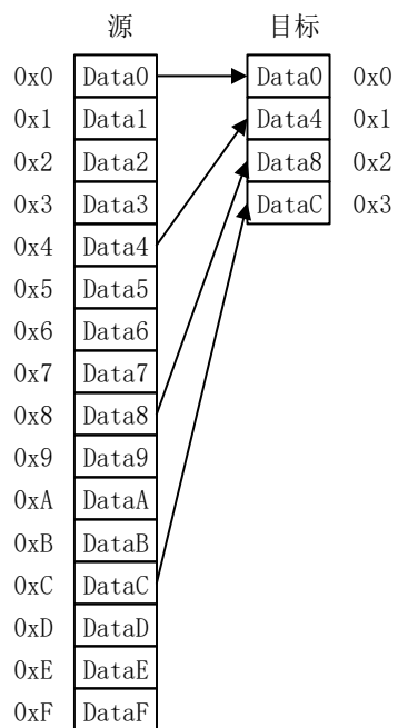
图 14 源为 32bits 目标为 8bits 的传输宽度
