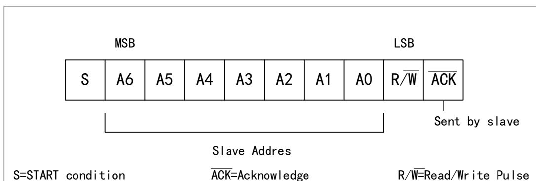
图 87 7 位地址格式
