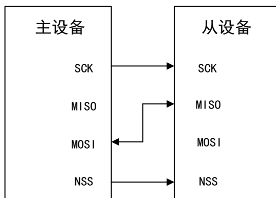
图 98 双向线连接
