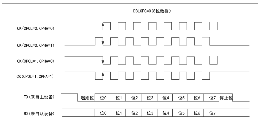
图 70 USART 同步传输时序图 (DBLCFG=0)
