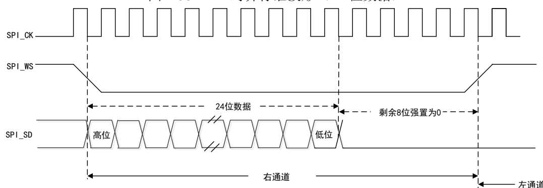
图 103 MSB 对齐标准波形（24 位数据）
