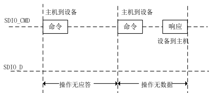
图 120 SDIO “无响应”和“无数据”操作
