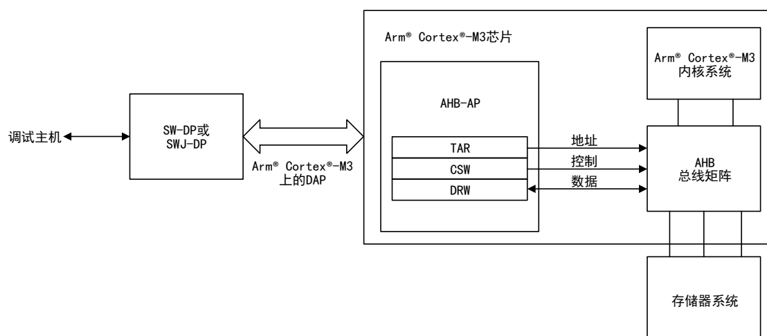
图 18 APM32E10xxx 级别和 Arm® Cortex®-M3 级别的调试框图
