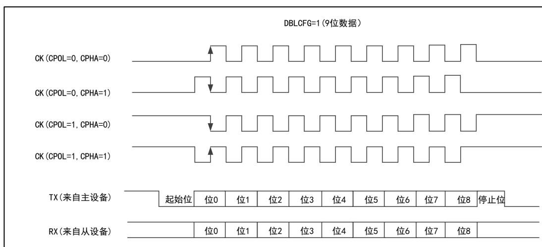
图 71 USART 同步传输时序图 (DBLCFG=1)
