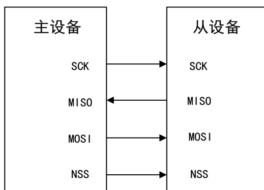
图 95 全双工模式连接
