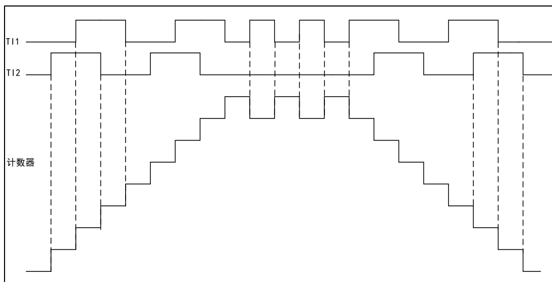
图 57 编码器模式下的计数器操作实例
