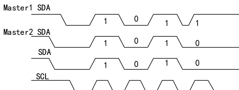
图 85 SDA 时序图
