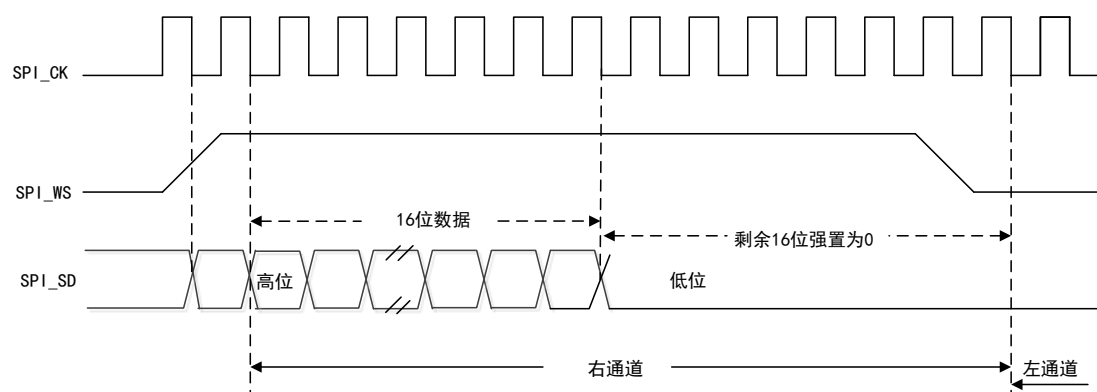
图 101 I2S 飞利浦协议波形（16 位扩展至 32 位）
