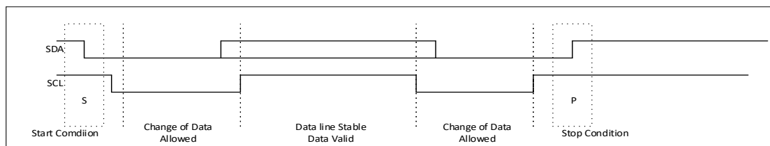
图 86 启动（START）和停止（STOP）条件
