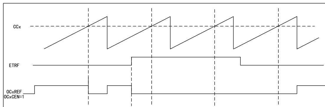
图 44 OCxREF 时序图
